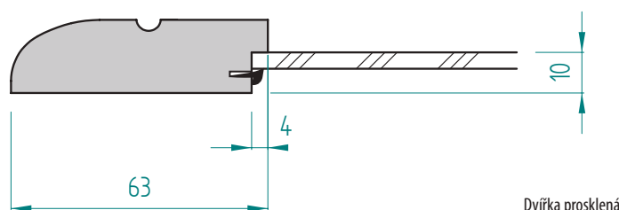
Dvířka prosklená
