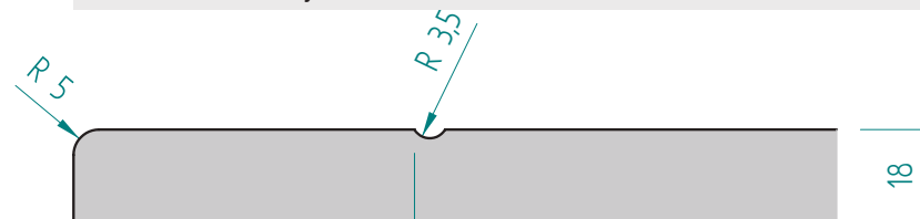
Dvířka plná
