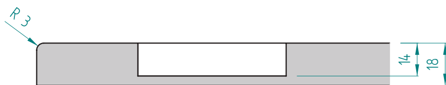
Dvířka plná
