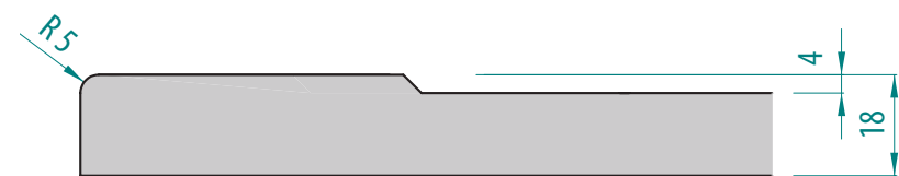
Dvířka plná
