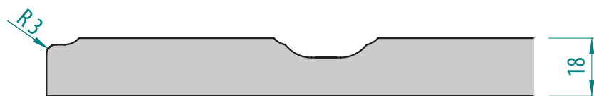
Dvířka plná
