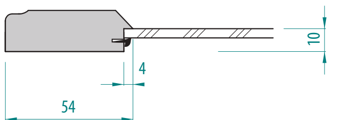
Dvířka prosklená
