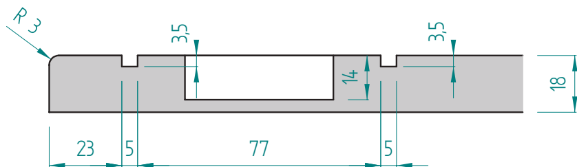
Dvířka plná
