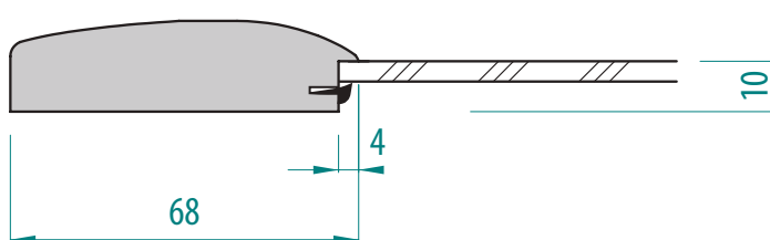
Dvířka prosklená
